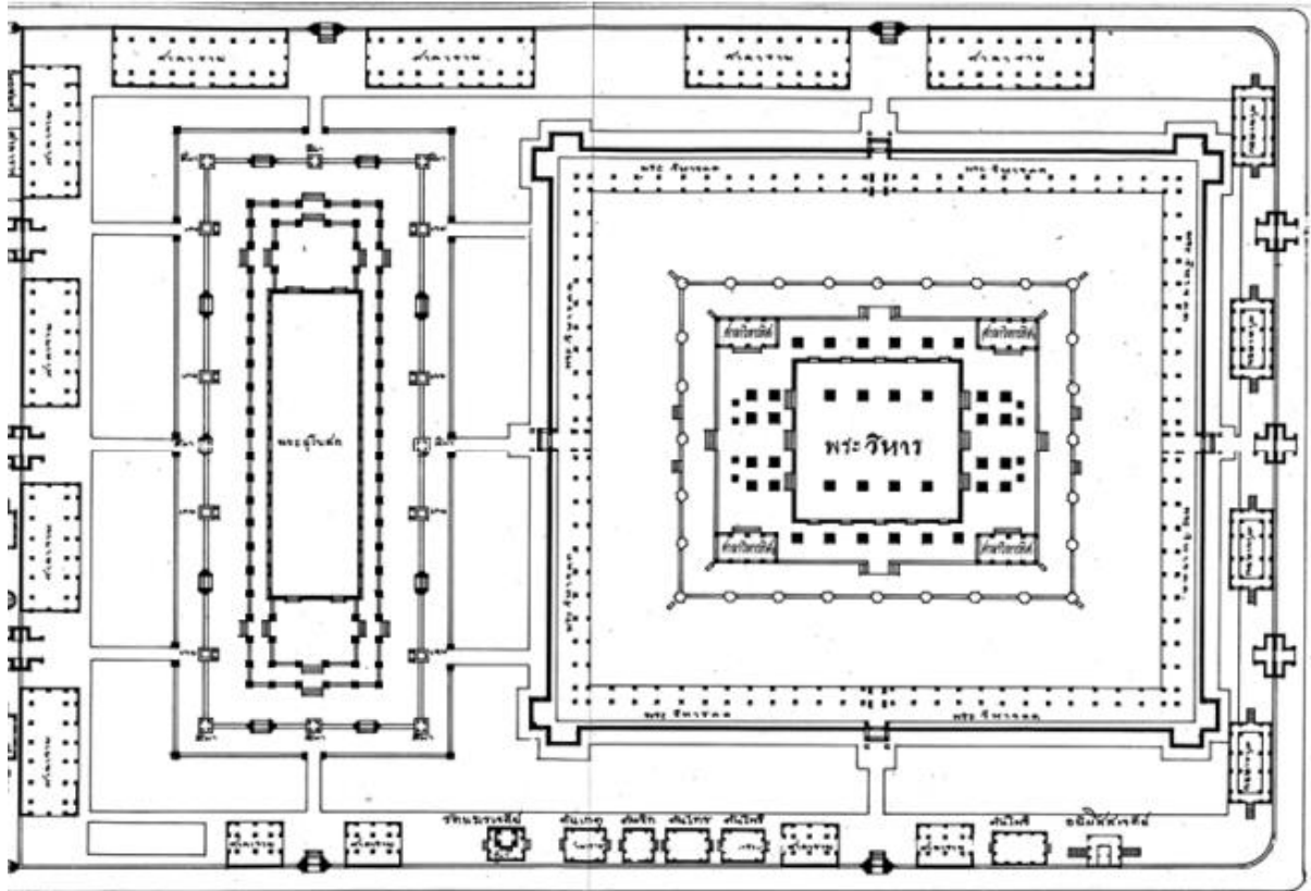
ผังวัดสุทัศนเทพวราราม แสดงรายละเอียดอาคารพระวิหารหลวง และอาคารพระอุโบสถ
